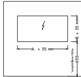
Einbaurahmen
