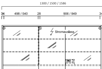
Spiegelschrank mit LED-Beleuchtung, Energieeffizienzklasse: A+, Tiefe 160 mm, Breite 1500 mm, LA0808... Breite 1586 mm, LA0808...
