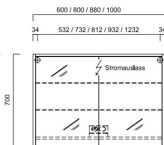
Spiegelschrank mit LED-Beleuchtung, Energieeffizienzklasse: A+, Tiefe 160 mm, Breiten: 600/800/880/1000 mm LA0808...
