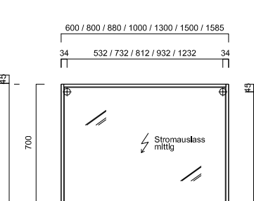
Lichtspiegel mit LED-Beleuchtung, Energieeffizienzklasse: A+, Breiten: 600/800/880/1000/1300/1500/1585 mm LA0808...
